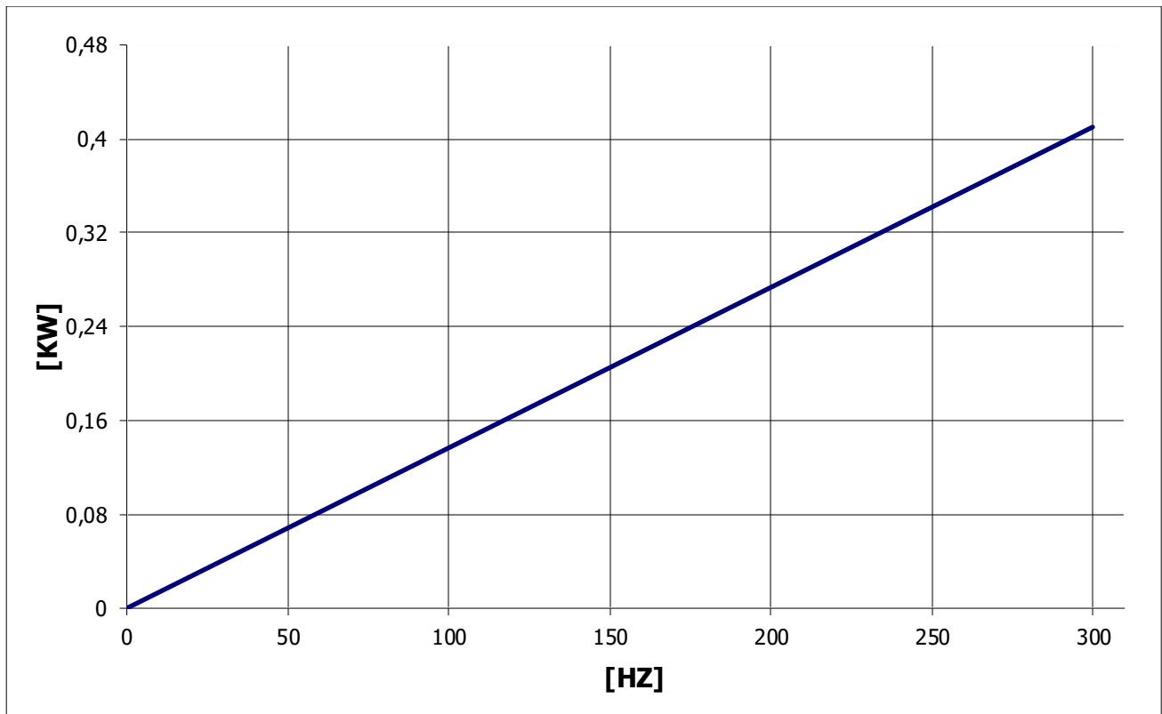
CURVA DI POTENZA - POWER CURVE
